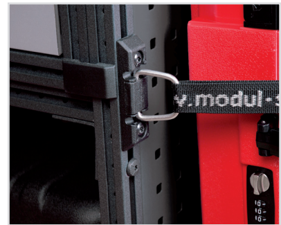
Befestigungsöse T-Nut Best. nr: 50025-03
